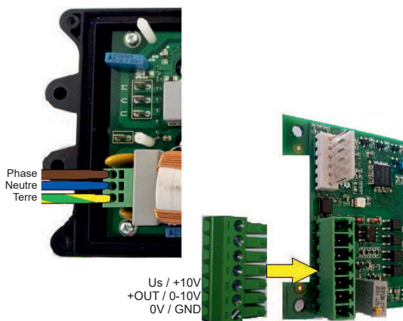
VMI 7/7-4 EC
