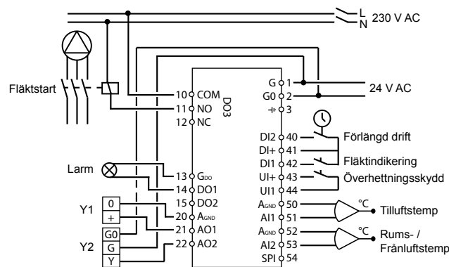
Figur 1. Inkopplingsexempel: OP10 med elvärme (till exempel via PULSER-X/D eller TTC25X) och spjäll. Kaskadreglering.
