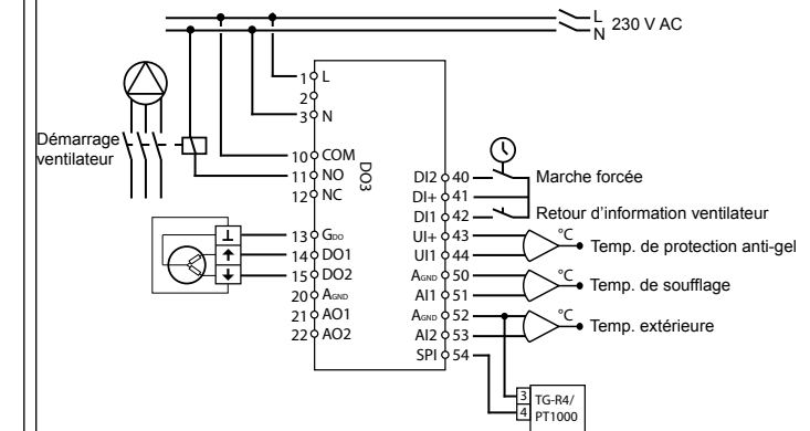
Figure 2. Exemple de câblage : OP10-230 pour batterie de chauffage à eau , sortie 3 points. Régulation du soufflage avec compensation de la température extérieure et potentiomètre de consigne externe.
