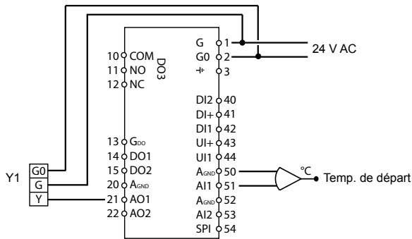
Figure 4. Exemple de câblage : OP10 avec moteur 0..0,10 V
