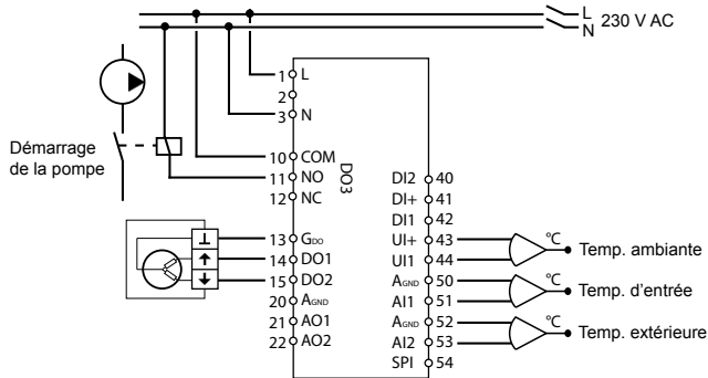
Figure 3. Exemple de câblage : OP10-230 avec moteur 3 points et sonde de température d'ambiance (s'utilise également sans sonde ambiante). Les sorties numériques ont une tension de 24 V AC, GDO est commun et DO est connecté à G0. Pour OP10, DO1 et DO2, les sorties acceptent du 12 VA. Pour OP10-230, DO1 et DO2, les sorties acceptent du 3,8 VA moyennant l'utilisation du transformateur interne.
