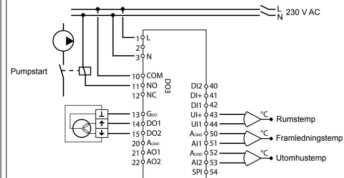
Figur 3. Inkopplingsexempel: OP10-230 med 3-lägesställdon och rumstemperaturlösgivare (kan även användas utan rumstemperaturlösgivare).
