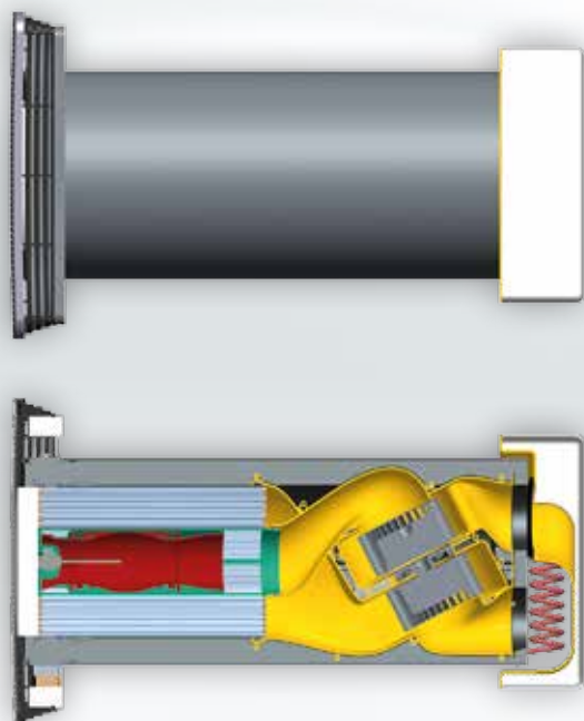
Dwarsdoorsnede Air 70
