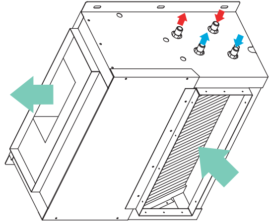
UNITA' ORIZZONTALE CON ATTACCHI IDRAULICI DESTRI HORIZONTAL UNIT WITH RIGHT HAND CONNECTIONS
