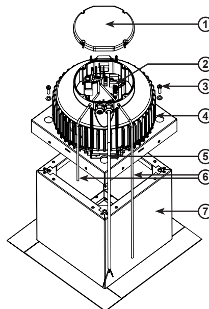
Fig. 2: Assembly size ARU-S...EC CP
