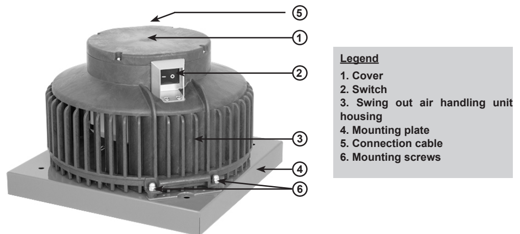
Fig. 1: Roof fan
