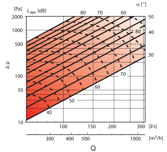
AKH Ø160
