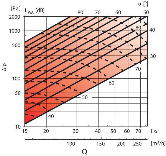
AKH Ø125
