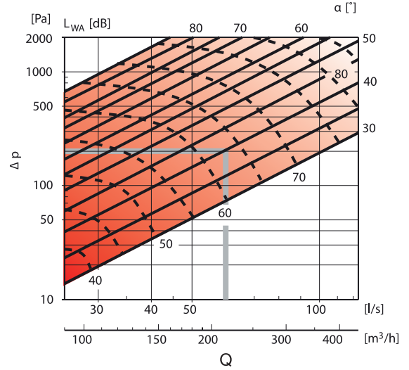
AKH Ø160
