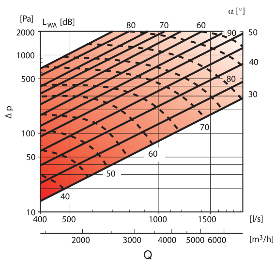
AKH Ø400
