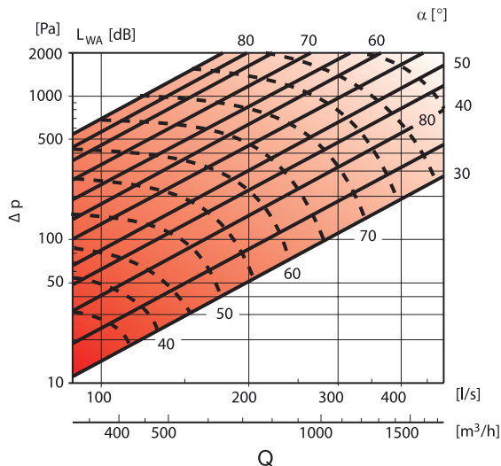
AKH Ø200
