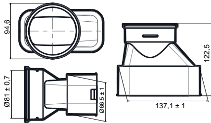
UDB-CON 60X130/55
