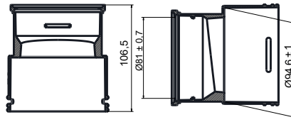
UDB-CON 50X100/35
