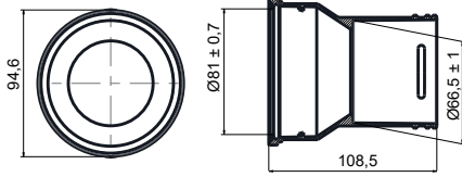
UDB-CON 60X130/55
