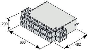
SKY 300 DB 160
