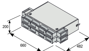
SKY 300 UDB 75
