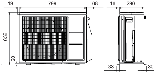
AOYG 24 KLTA
