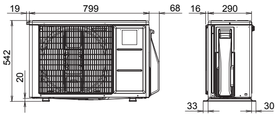
AOYG 18 KLTA
