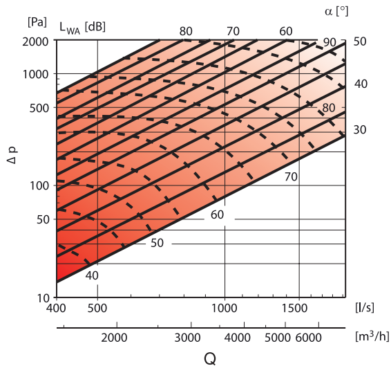
AKH Ø400
