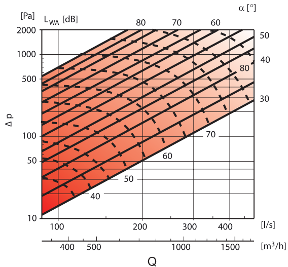
AKH Ø200
