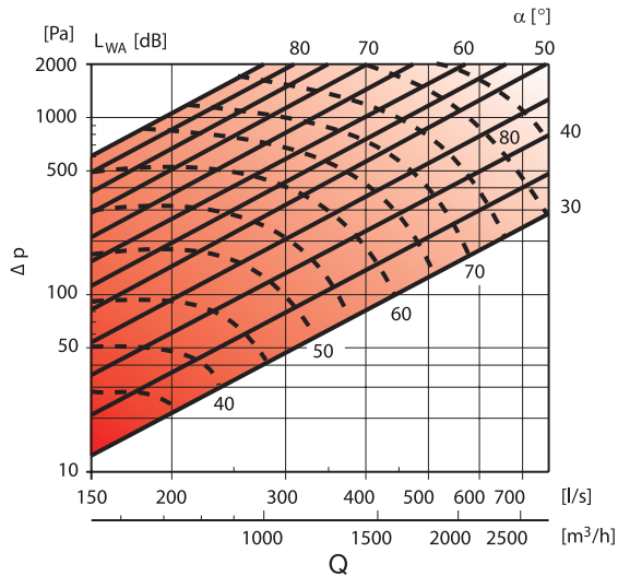
AKH Ø250
