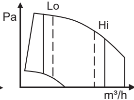
Hexamotion QUATTRO EC
