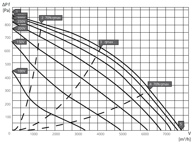
ARFV-S 500 D4 30
