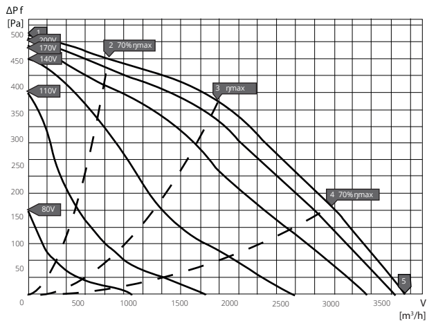
ARFV-S 500 D4 30
