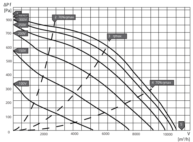
ARFV-S 560 D4 30
