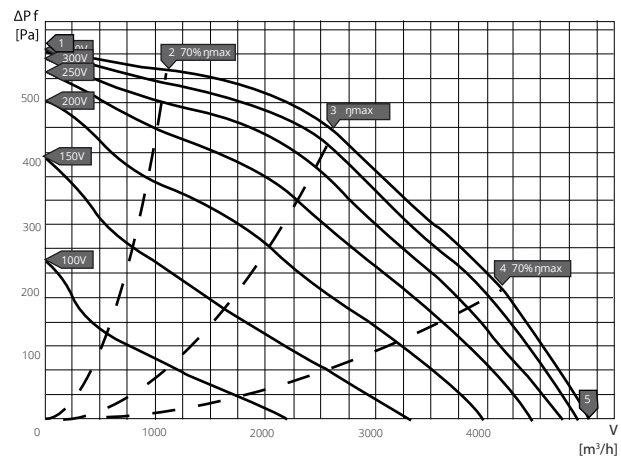
ARFV-S 560 D4 30
