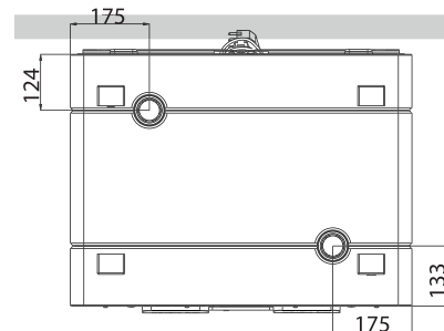
Onderaanzicht Vue de dessous
