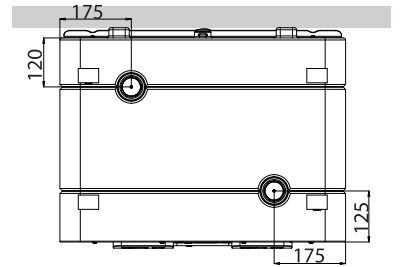
Onderaanzicht Vue de dessous
