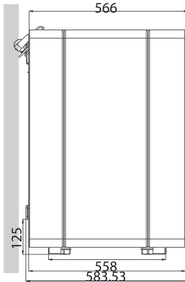
Zij-aanzicht Vue latérale
