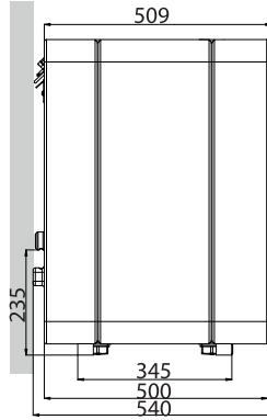
Zij-aanzicht Vue latérale
