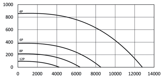
RFV-P 63/3
