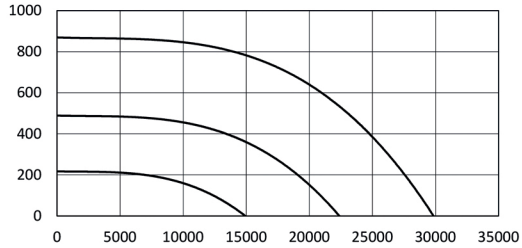
RFV-P 80/4
