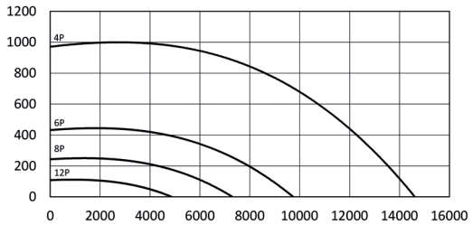
RFV-P 71/4
