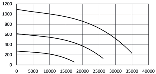
RFV-P 90/4
