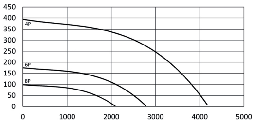
RFV-P 50/2
