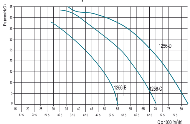
DUCT-M 1250 - 6 poles
