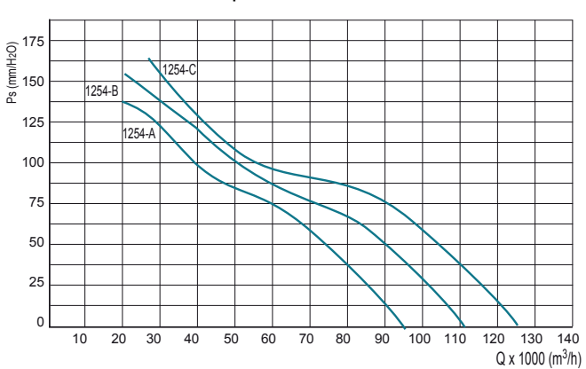
DUCT-M 1250 - 4 poles
