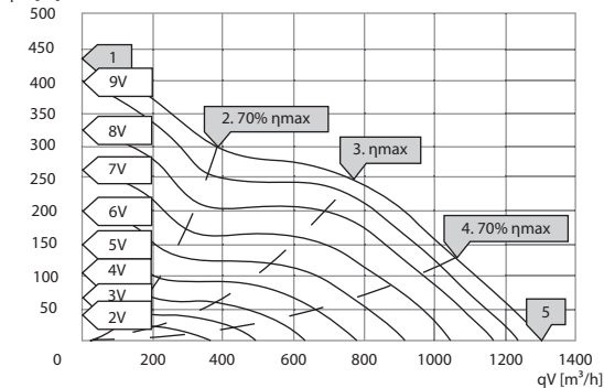
ETAMASTER 200L EC 01
