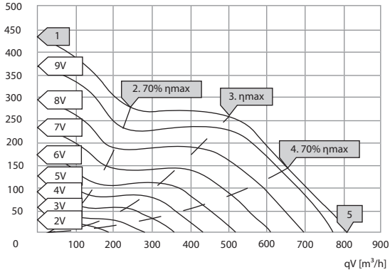
ETAMASTER 160L EC 01
