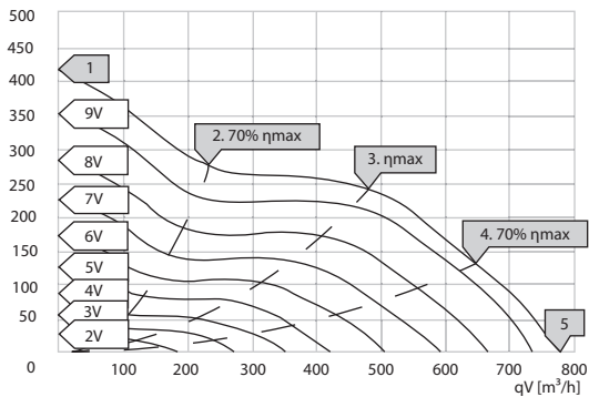
ETAMASTER 150L EC 01
