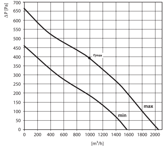
TT MIX PRO 315
