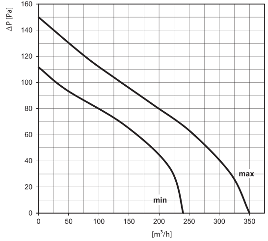
TT MIX PRO 125
