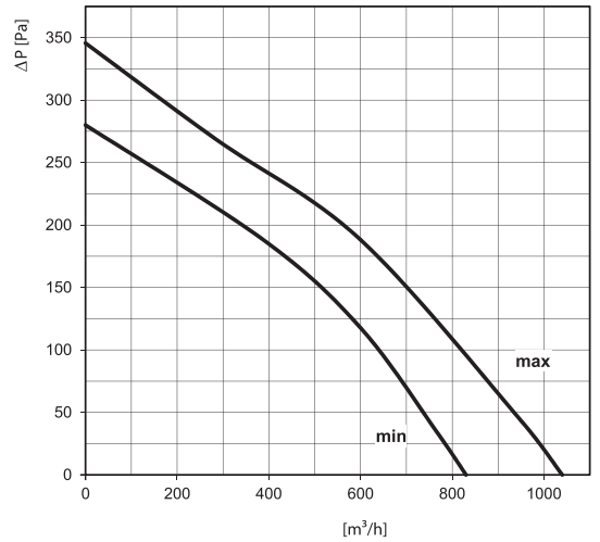
TT MIX PRO 200
