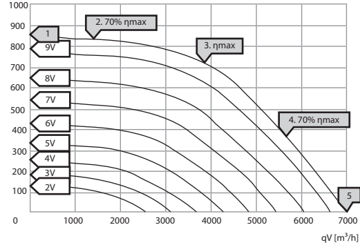
psf [Pa] KBF-N 630 D4 T30
