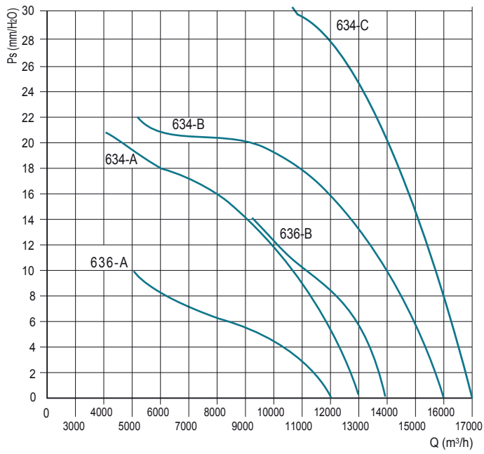
DUCT-M 800 - 4 poles
