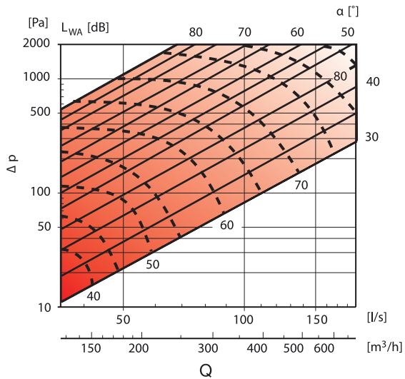
KDM Ø125
