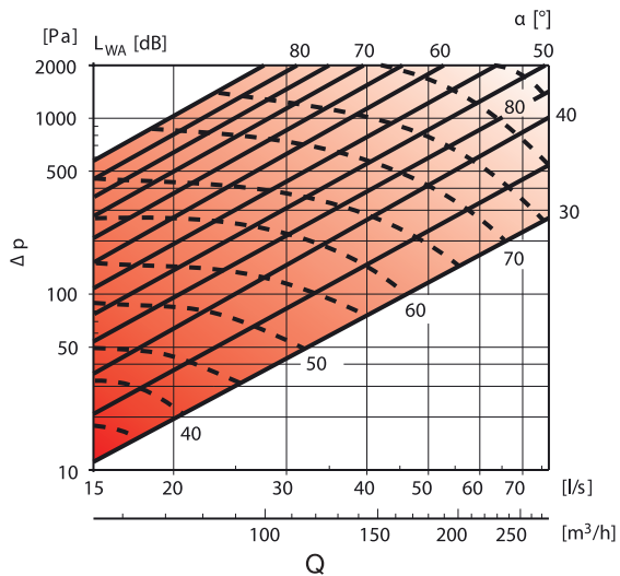
KDM Ø125
