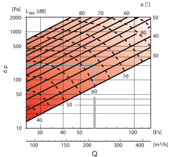
KDM Ø160
