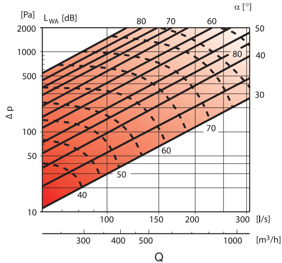
KDM Ø160
