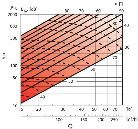
AKH Ø125
