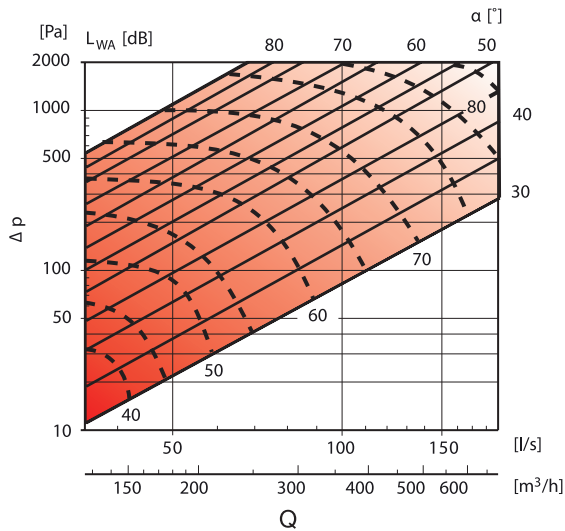
AKH Ø125
