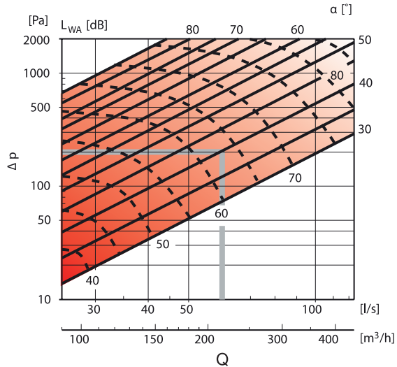
AKH Ø160
