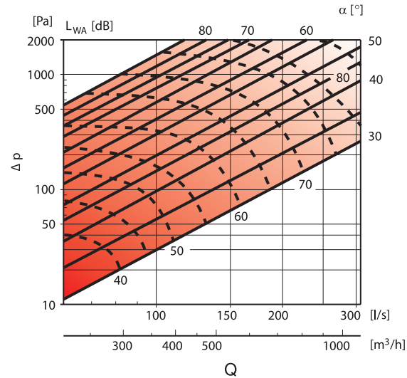
AKH Ø160
