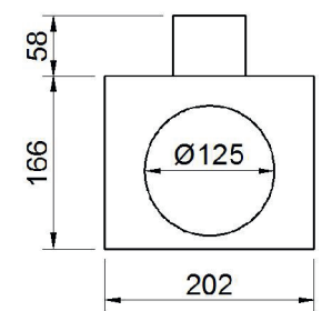
S-COL C 125/1x70
