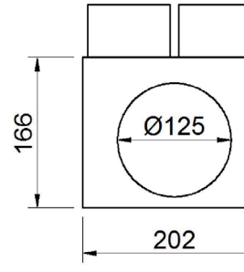
S-COL C 125/2x90
