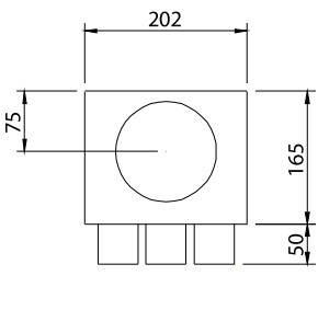
S-COL C 125/5x50
