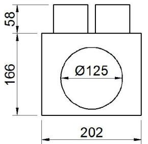
S-COL C 125/2x70
