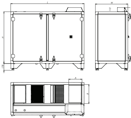
AmberAir Compact 1-5 CXV
