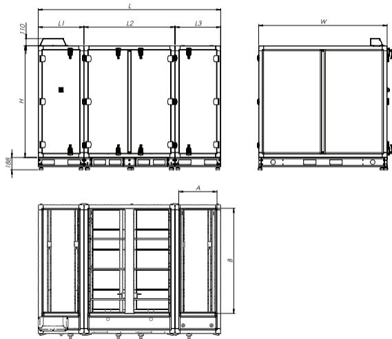
AmberAir Compact 6-7 CXV
